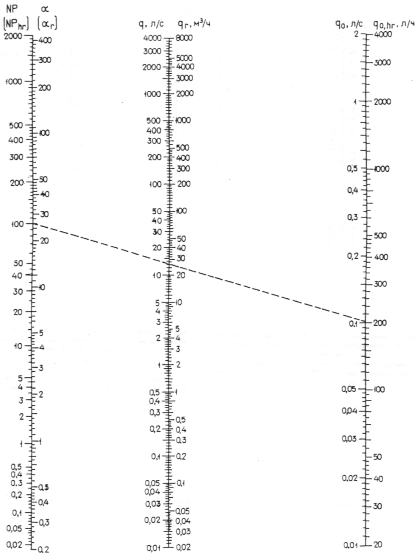
Черт.4. Номограмма для определения секундных и часовых расходов воды в зависимости от NP ( NP_{hr} ) при различных значениях q_0 , л/с, q_0, \text{hr} , л/ч
