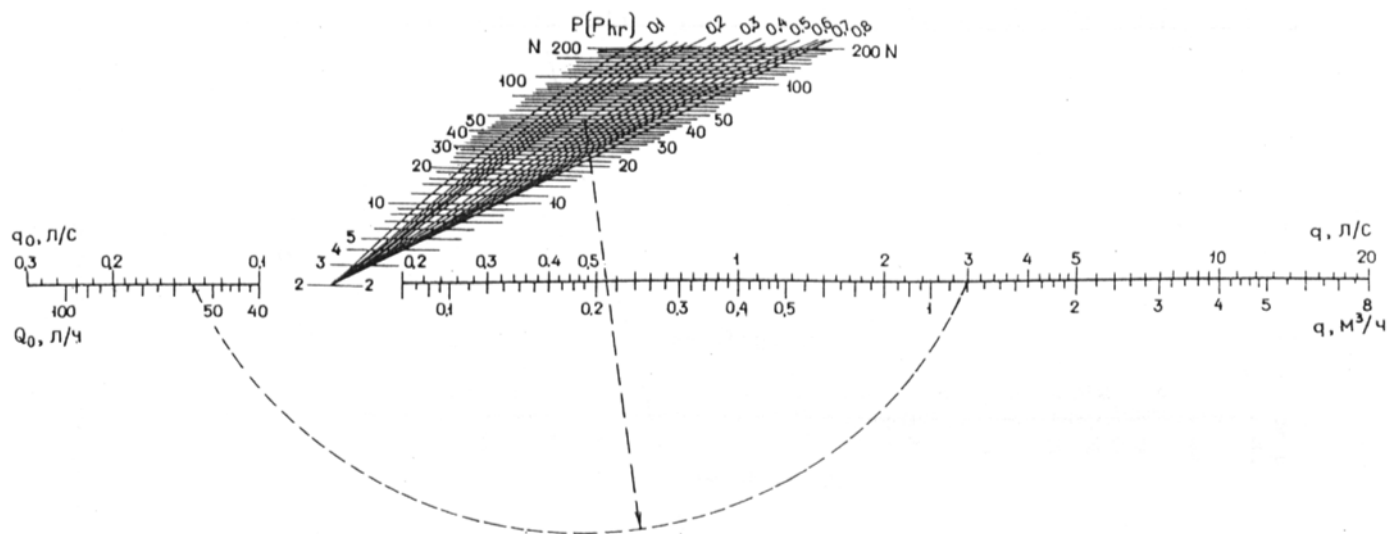
Черт.2. Номограмма для определения секундных расходов воды q при q_0 = 0,2 и 0,3 л/с и P \leq 0,15
