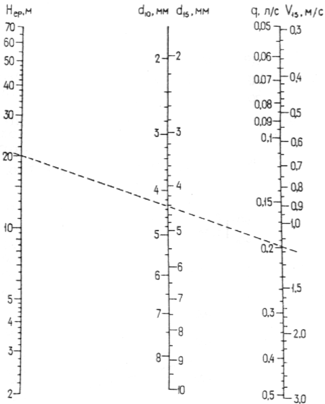
Черт.6. Номограмма для определения диаметров отверстий диафрагм, устанавливаемых у смесителей водоразборной арматуры санитарных приборов d_{10} ( d_{15} ) - диаметр отверстия
